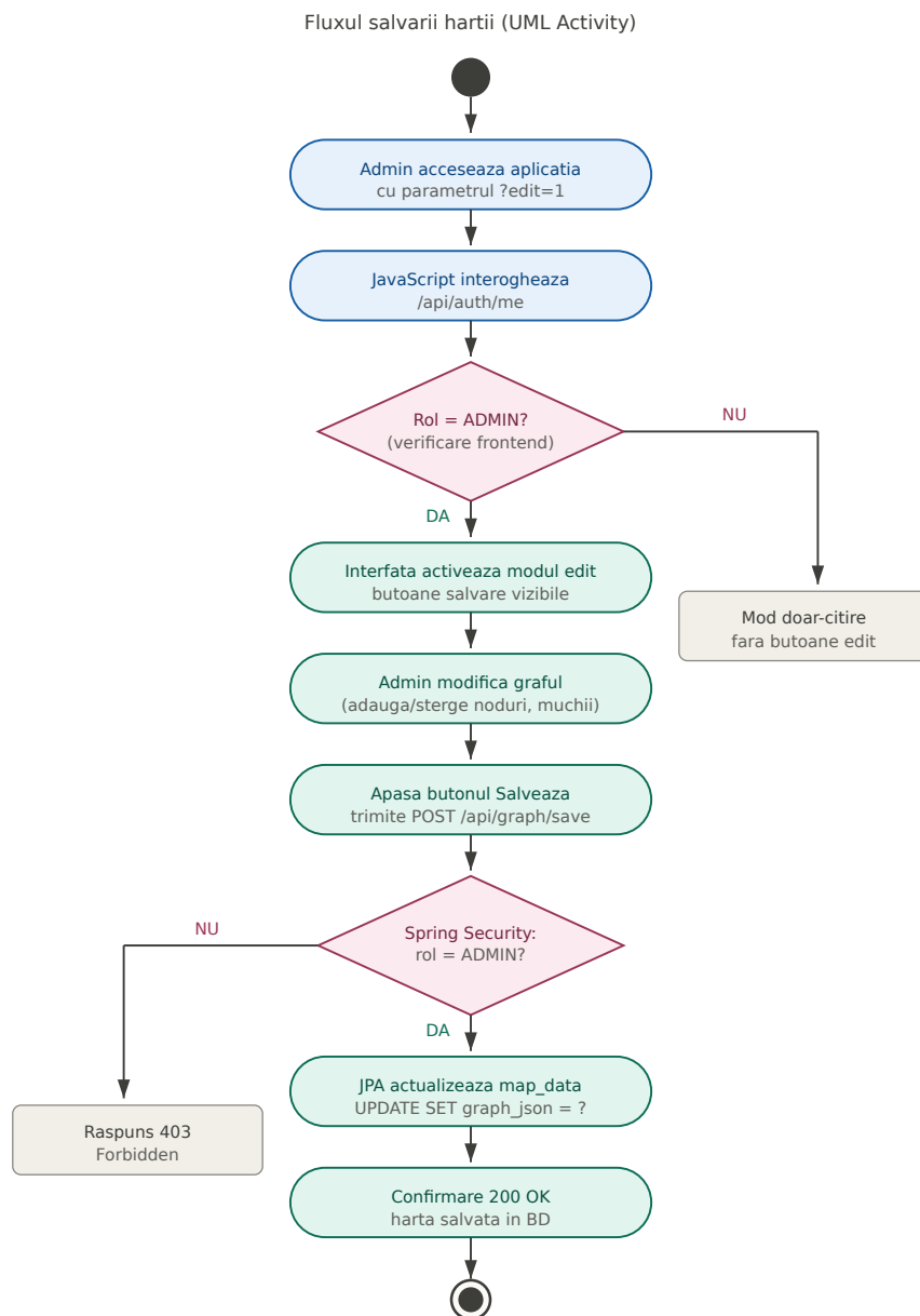
Figura 3.4: Diagrama UML de activitate care prezintă fluxul de editare și salvare a hărții.
